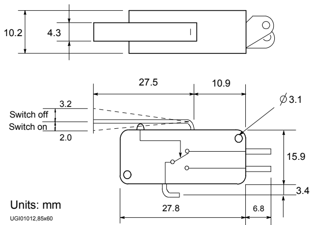
Figure 3-10 インターロック・スイッチの寸法 (Agilent 部品番号 3101-3241)
